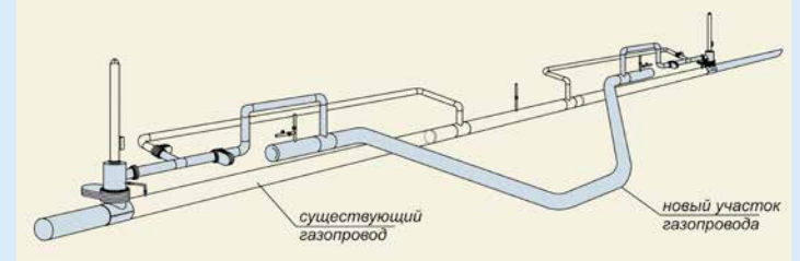
Схема врезки под давлением обводного участка газопровода-отвода Ду-500
